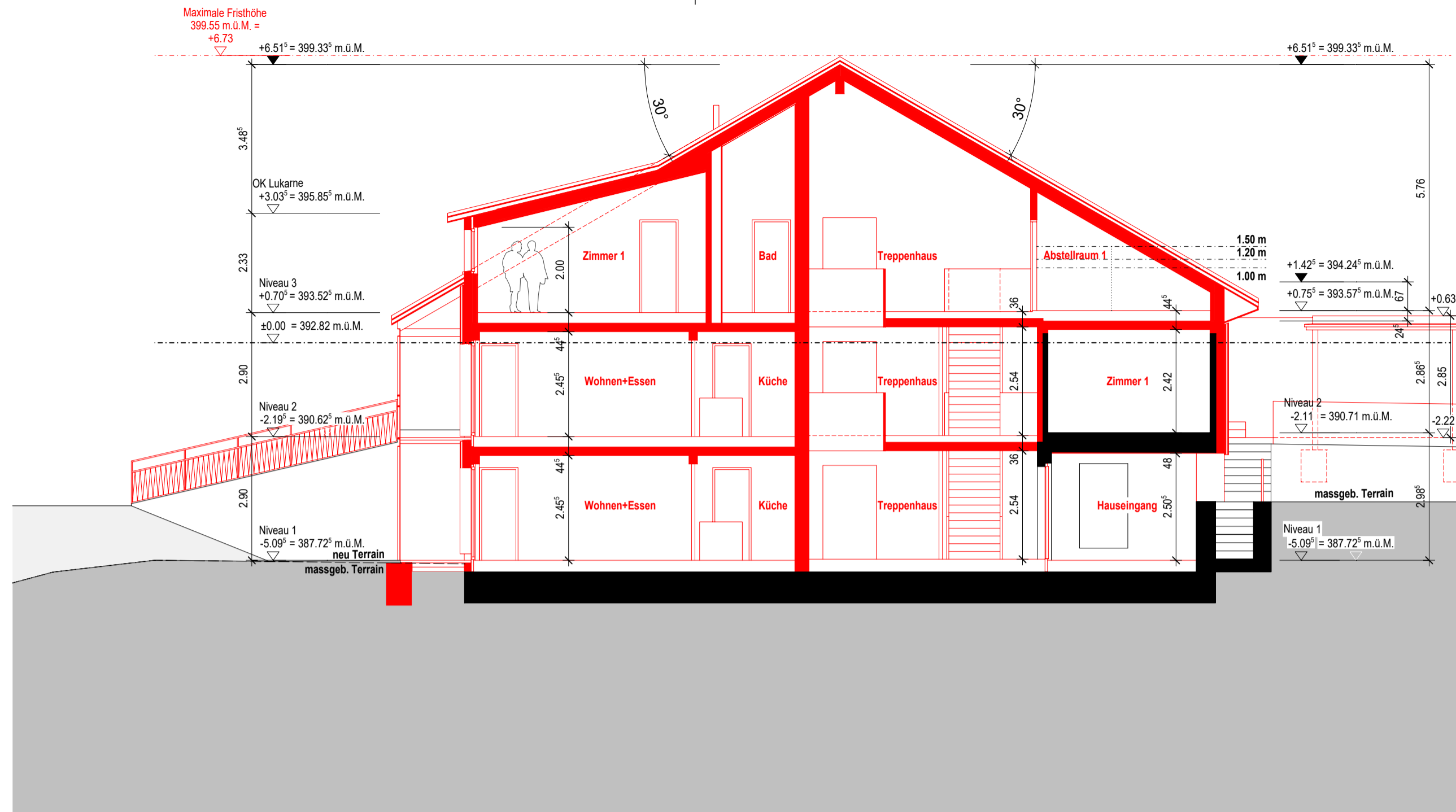
SCHNITT F
