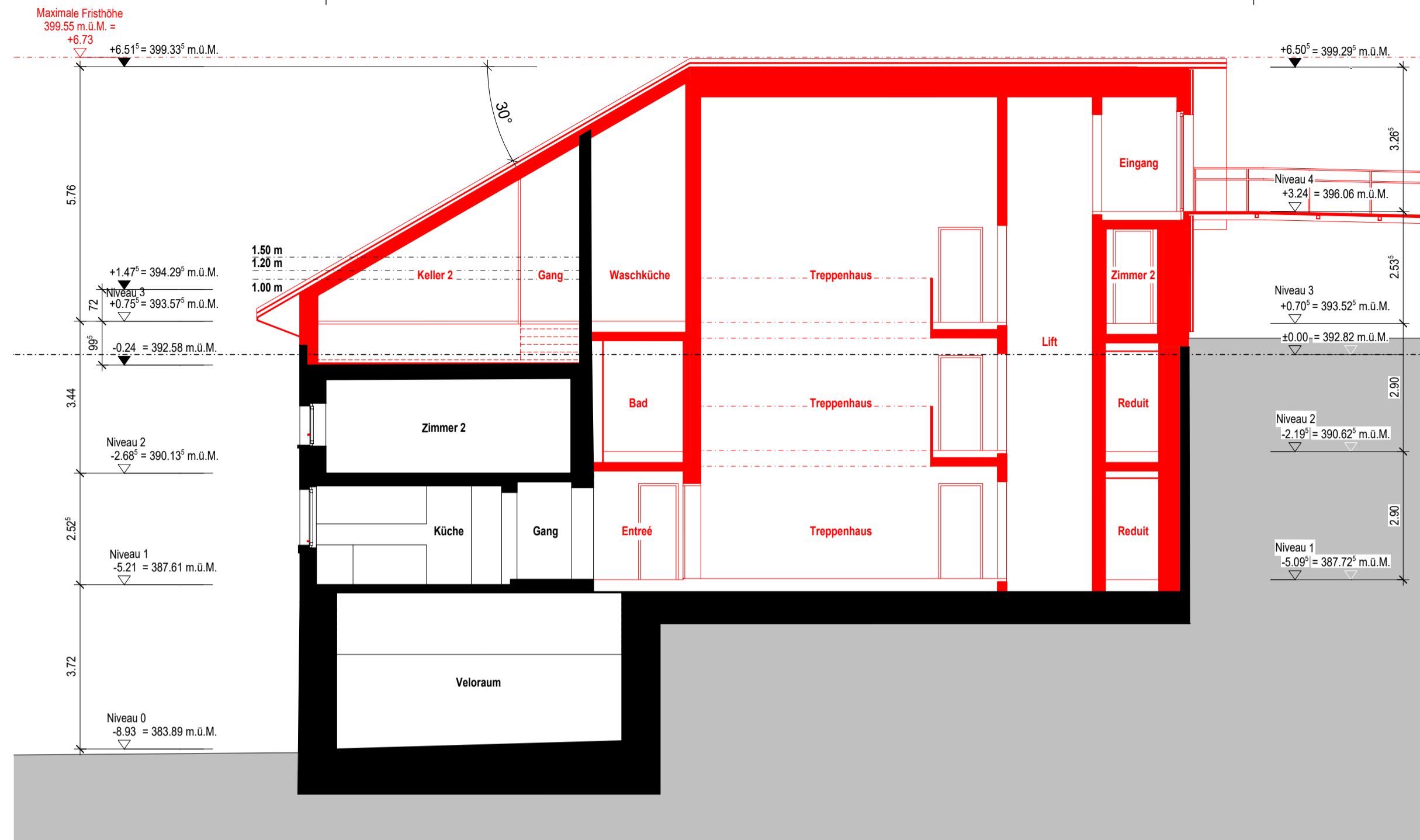
SCHNITT E
