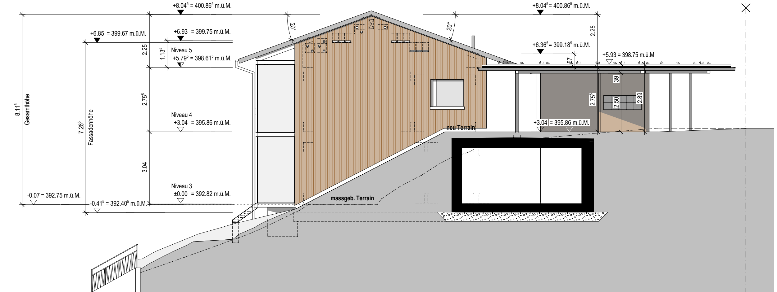
OSTFASSADE
