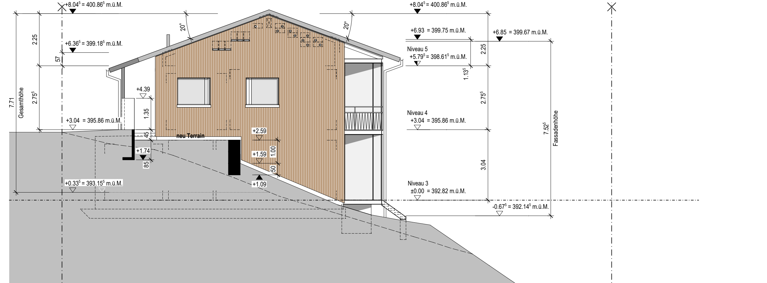
WESTFASSADE
