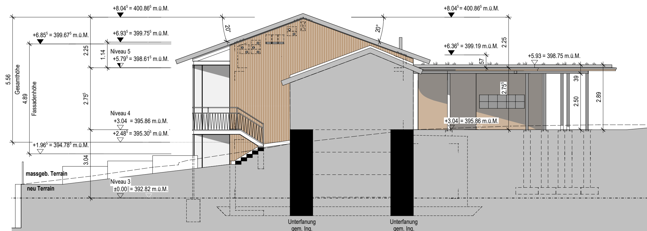
OSTFASSADE
