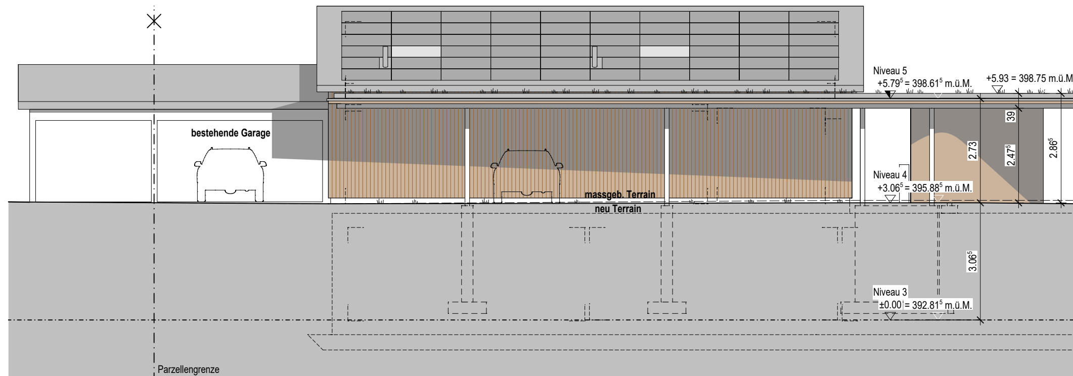
NORDFASSADE
