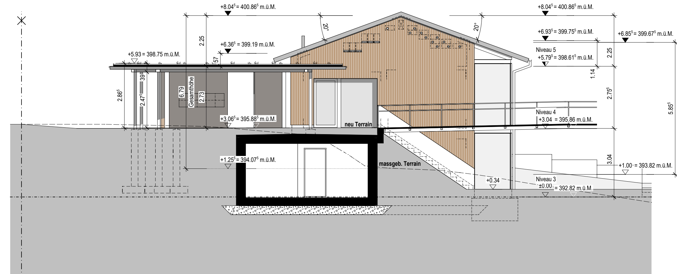
WESTFASSADE
