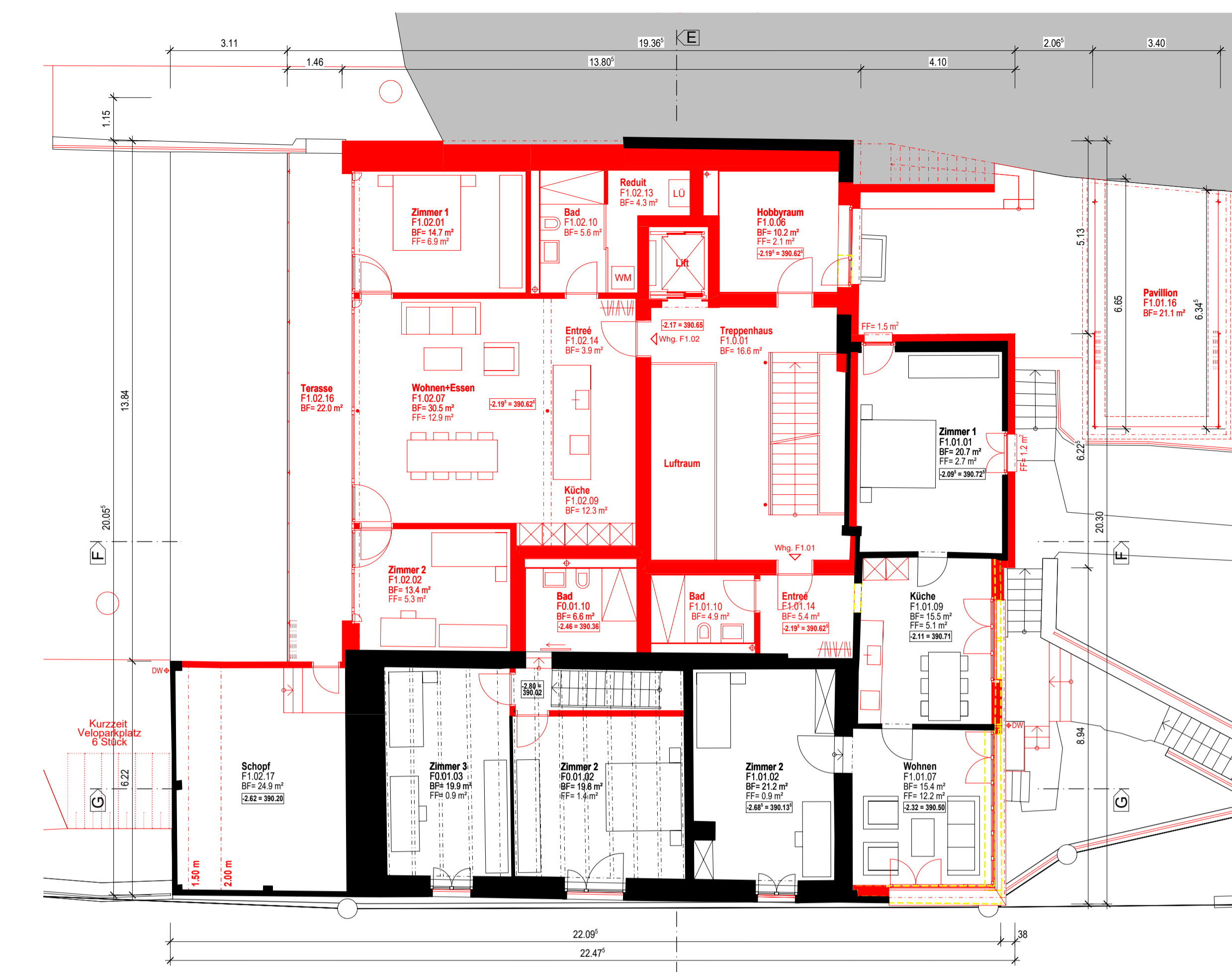
NIVEAU 2
