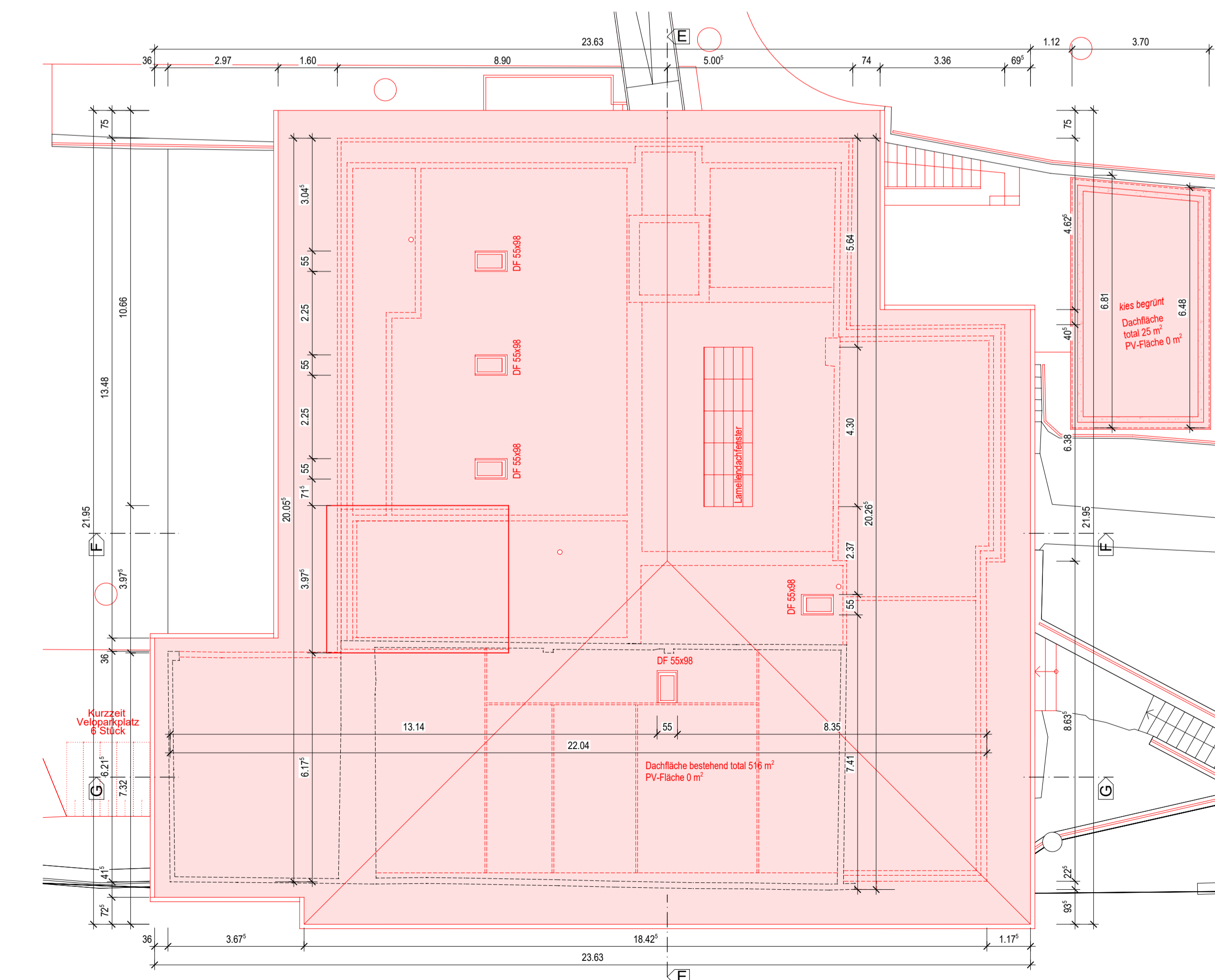
DACHAUFSICHT
