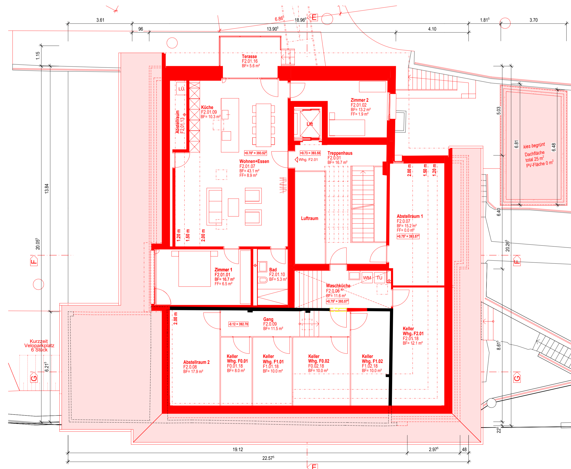
NIVEAU 3
