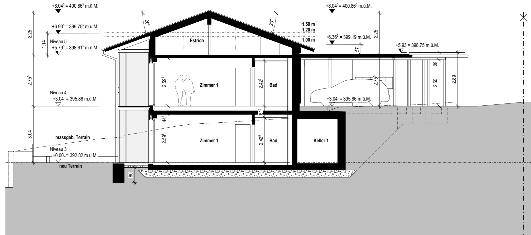
SCHNITT A-A
