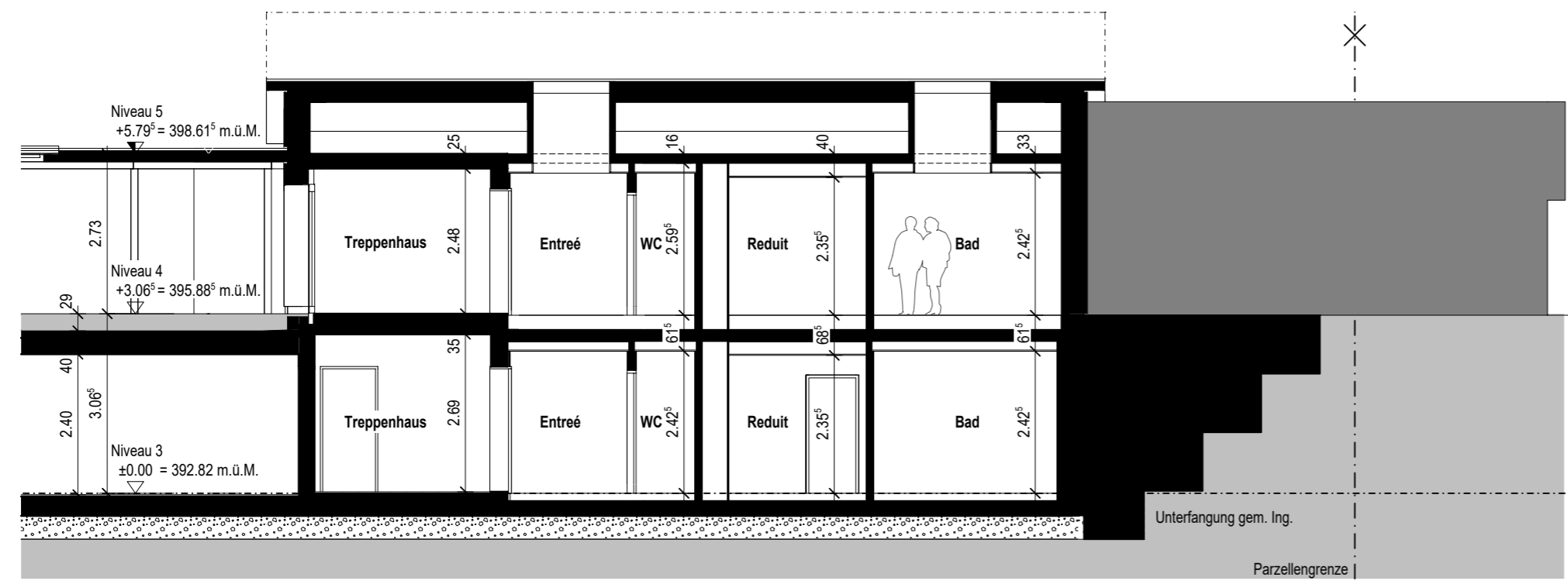
SCHNITT B-B
