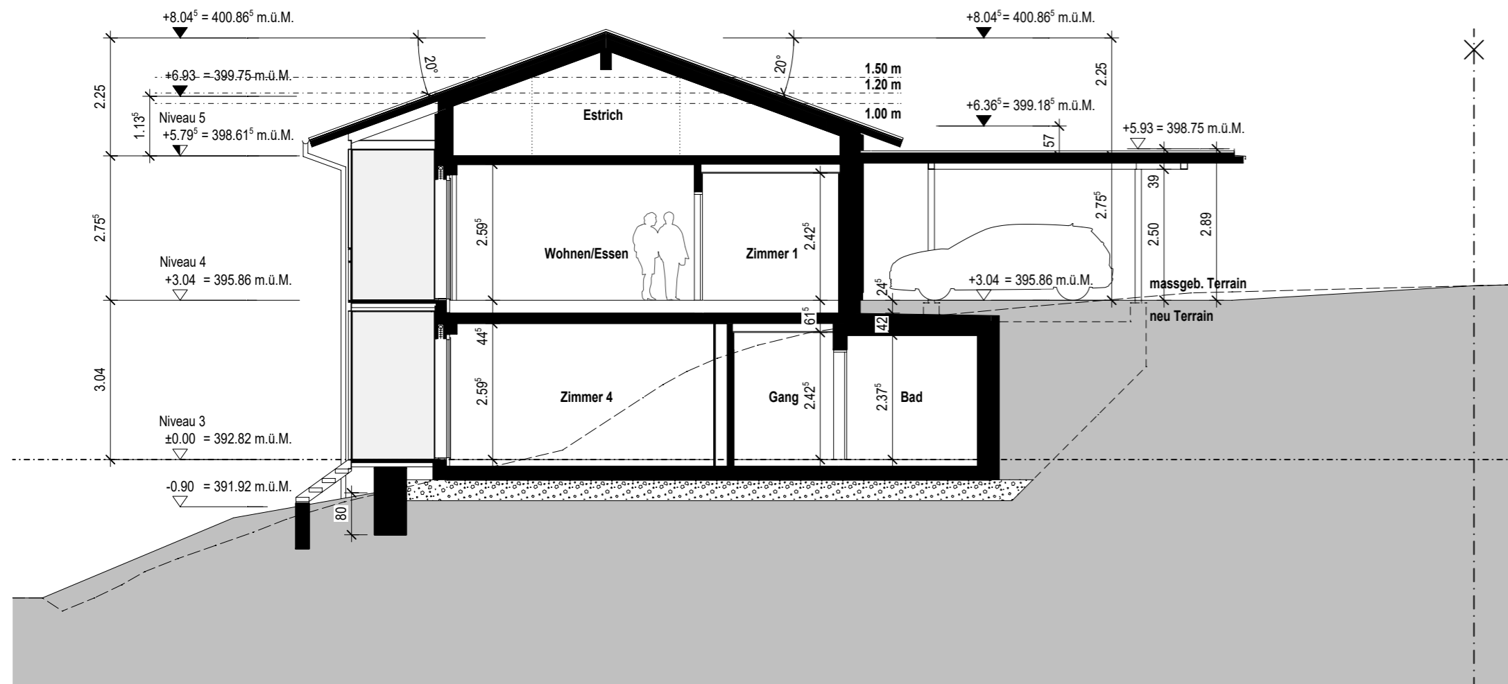
SCHNITT C-C
