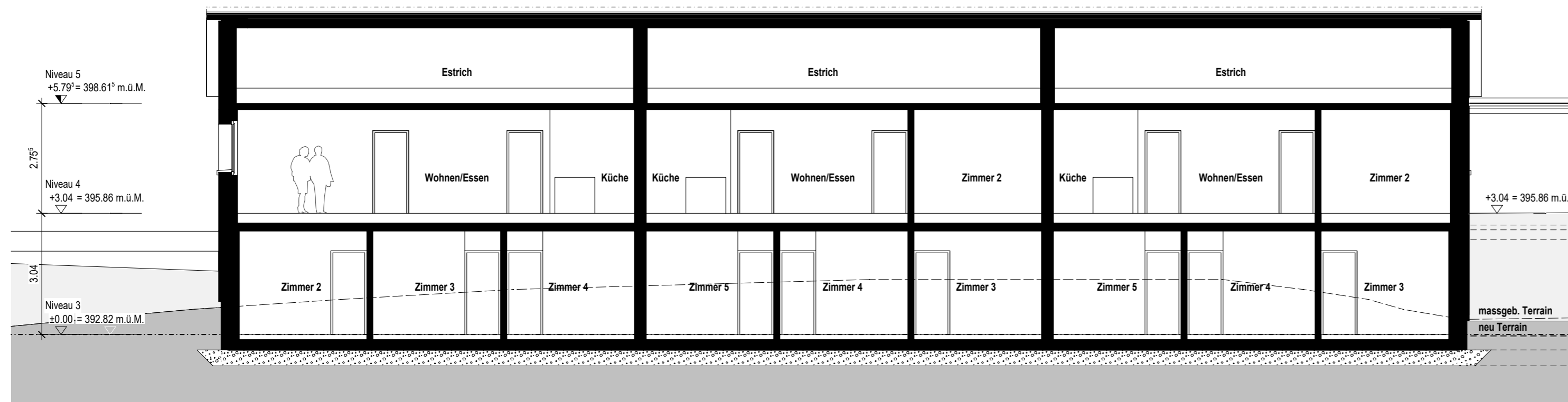
SCHNITT D-D
