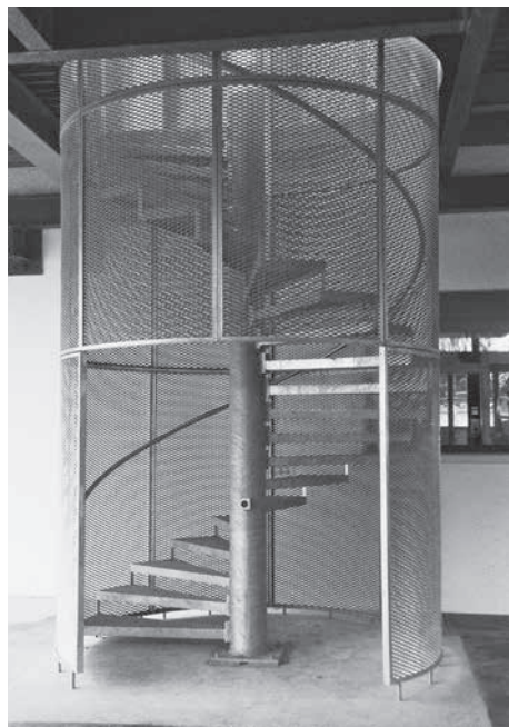
Spindeltreppe mit Streckmetall Einfassung.
